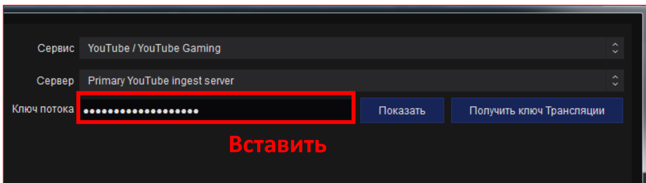
Рисунок 8 – Настройка вещания.
