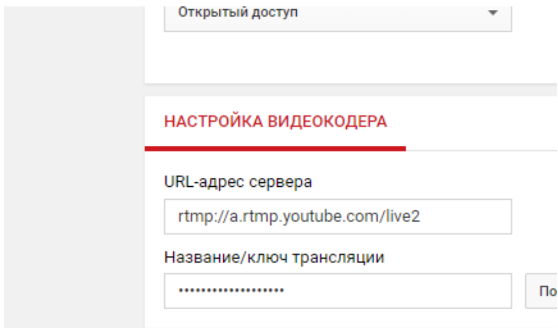
Рисунок 6 – Ключ трансляции
