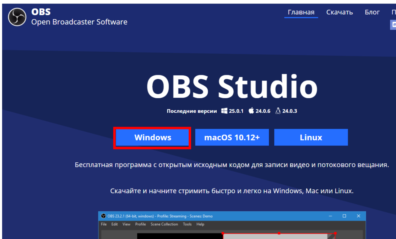
Рисунок 1 – Главная страница
