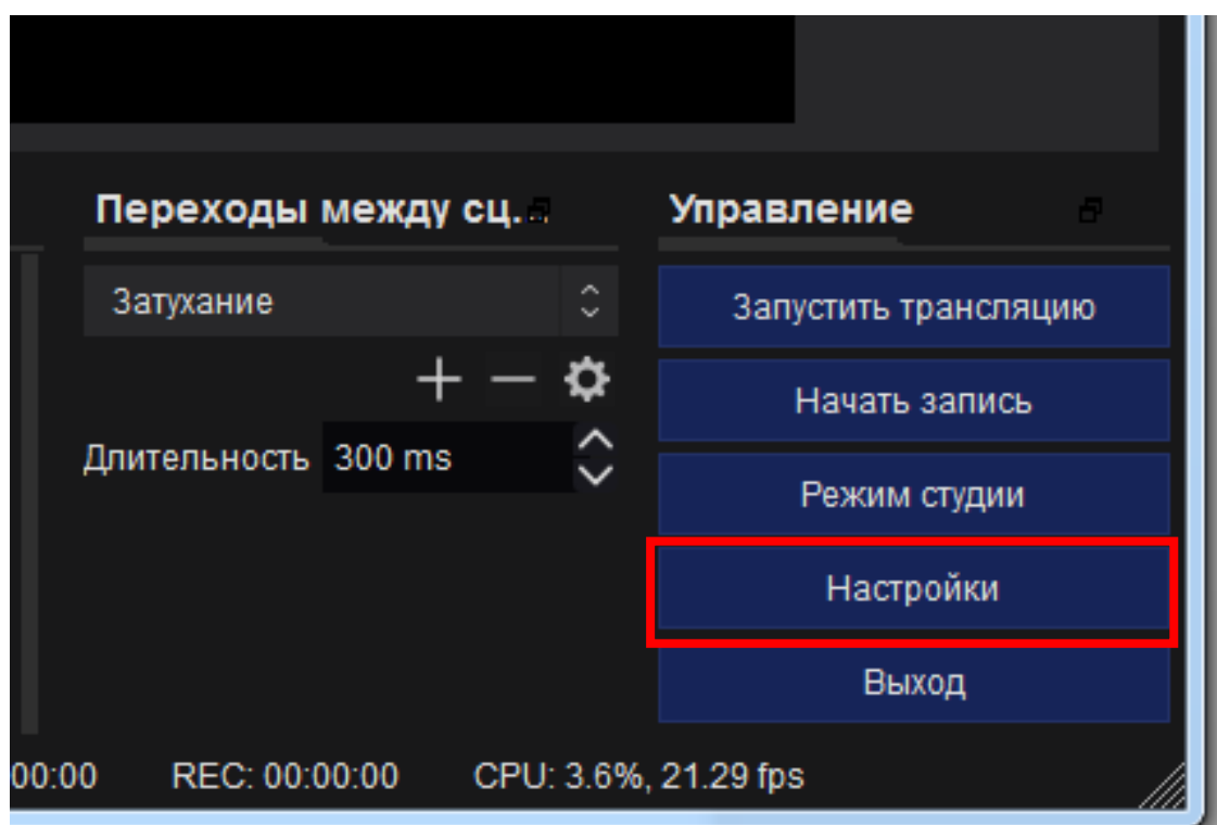
Рисунок 7 – Настройка OBS
