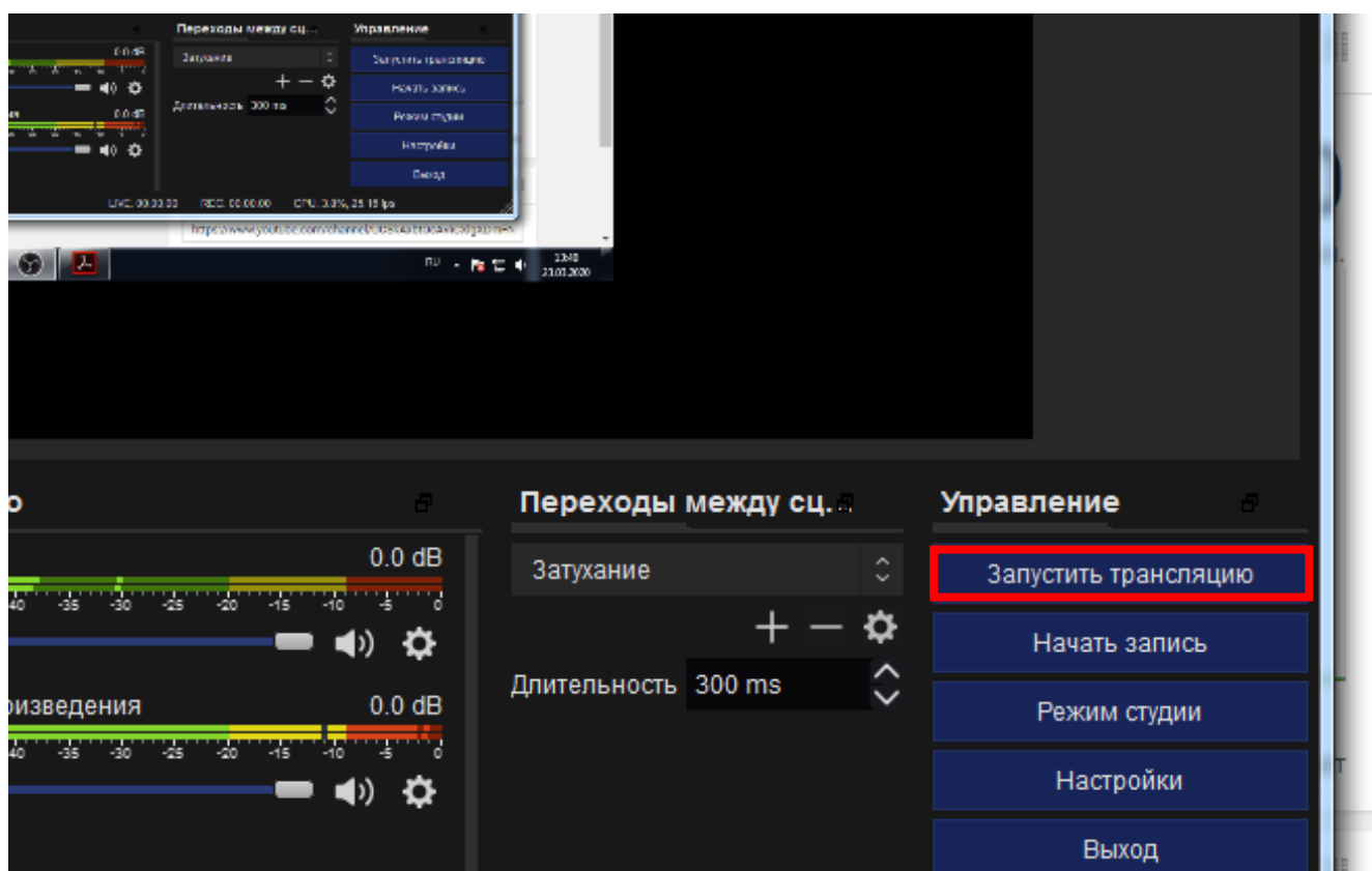
Рисунок 9 – Запуск трансляции
